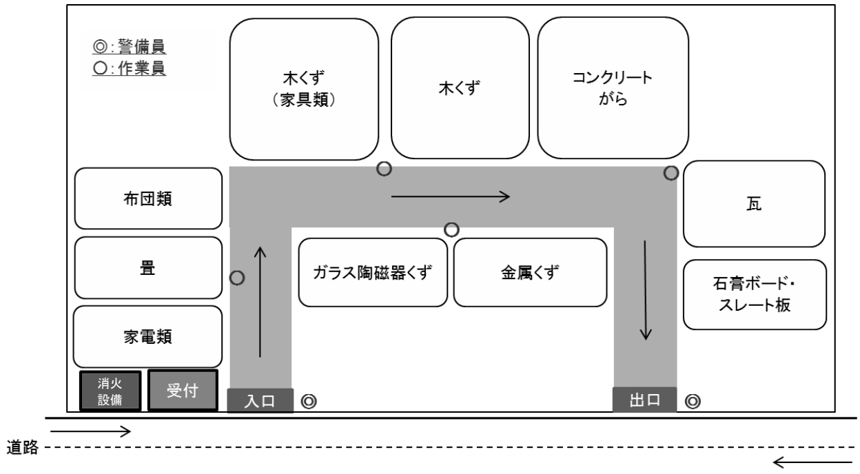
図2-6-5 仮置場の分別配置の例
